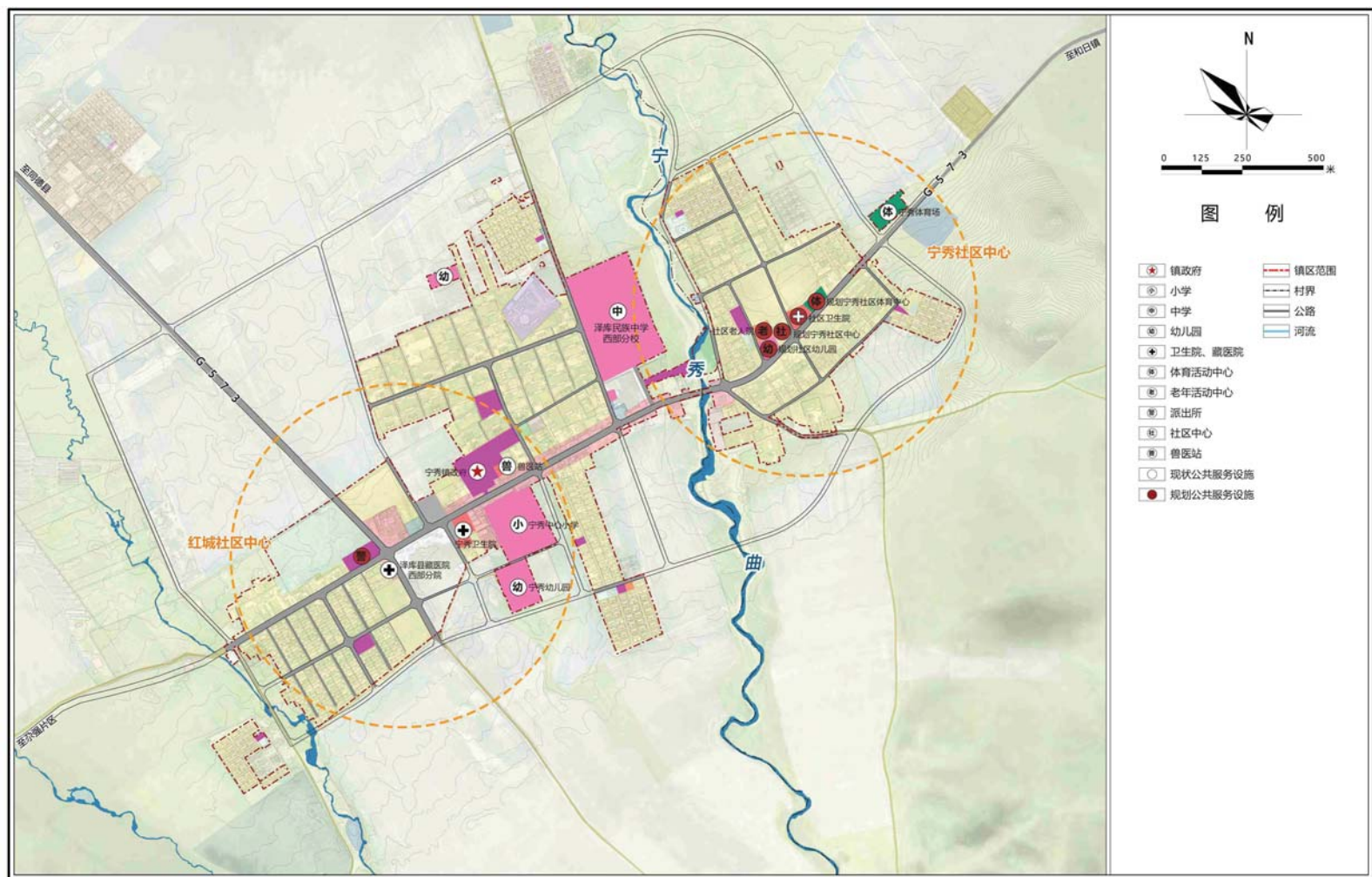
镇区公共服务设施布局规划图
